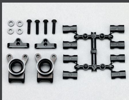
アルミ製 リヤハブキャリア (φ3 ピン)
