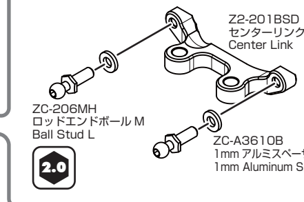
ZC-206MH ロッドエンドボール M Ball Stud L
