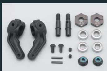
六角ホイールハブ/ ST ブロックコンバージョンキット B2-HCOV ¥1,980
