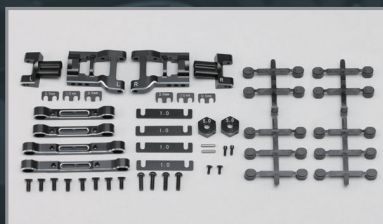
YD-2 シリーズ 用 アップグレード 3 アルミ 可変リアサスマーム セット
