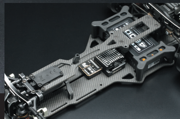
バッテリーを最後方に設置し、リヤトラクションを最大限に高めるウエイトバランス
