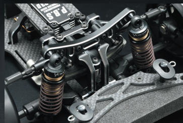
アルミ製一体型バルクヘッド、グラファイト製バンパーなど、最新のオプションを標準装備
